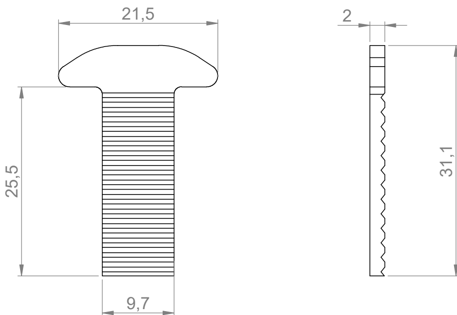
DIMENSÕES (SEM ESCALA)
