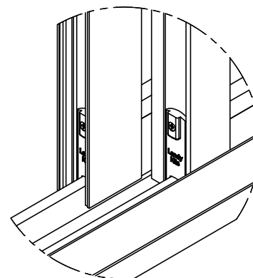
DETALHE A FIXAR 2 PEÇAS EM CIMA E DUAS EM BAIXO NA LATERAL DE CADA FOLHA, TOTALIZANDO 4 PEÇAS POR FOLHA
