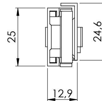
DIMENSÕES (ESCALA 1:1)
